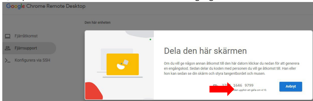
Figur 3: Kopiera koden
